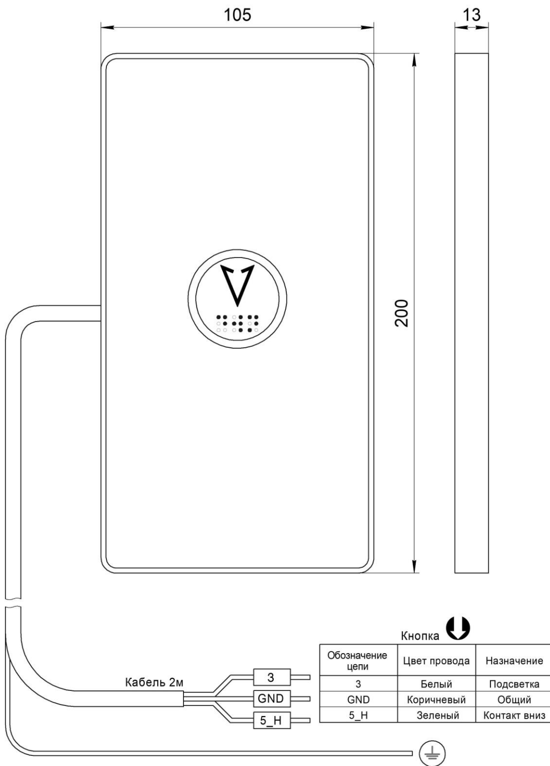
Рис.1 Внешний вид и габаритные размеры Вызывного поста МАЛАХИТ НШЕК.468381.062
