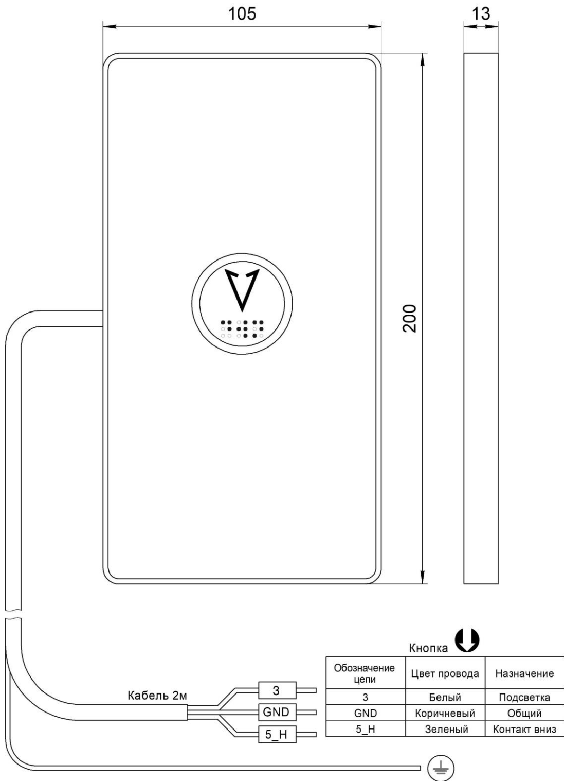
Рис.1 Внешний вид и габаритные размеры Вызывного поста МАЛАХИТ НШЕК.468381.062
